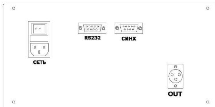
Рисунок 3. Внешний вид задней панели
