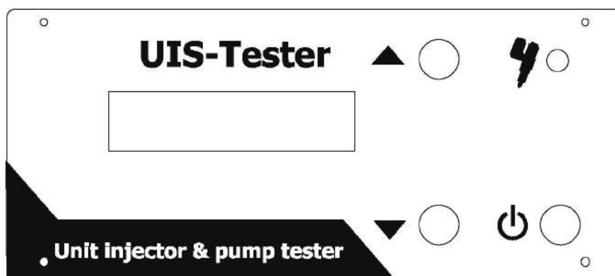
Рисунок 2. Внешний вид передней панели
