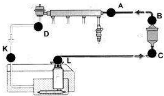
Система L- JETRONIC/ MOTRONIC с топливным электронасосом, установленном в топливном баке
