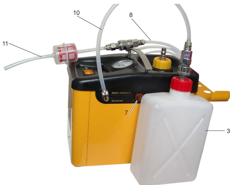
Рисунок 3. Режим «Откачка»
