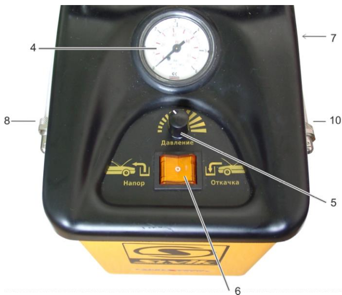
Рисунок 2 - Органы управления
