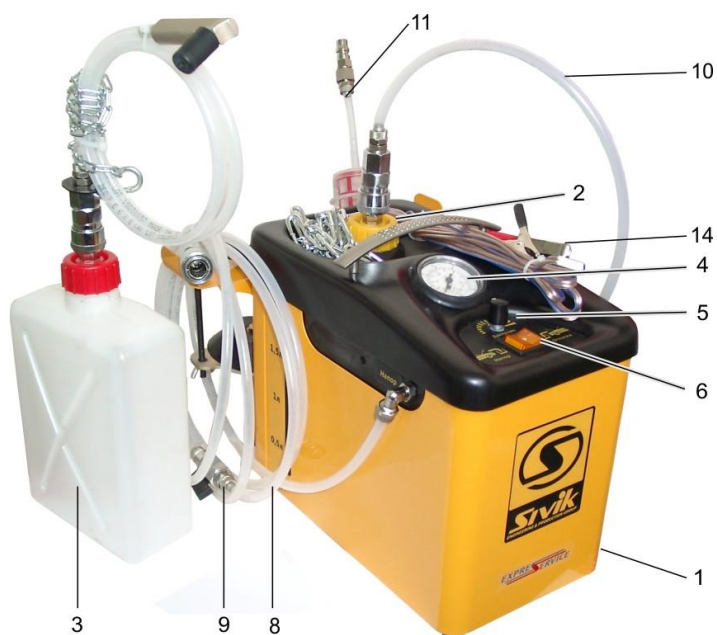
Рисунок 1 - Внешний вид установки
