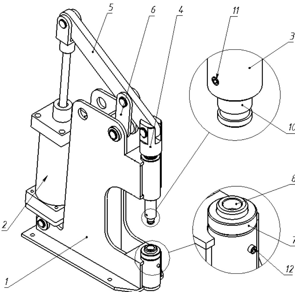
Рис. 2. Устройство станка
