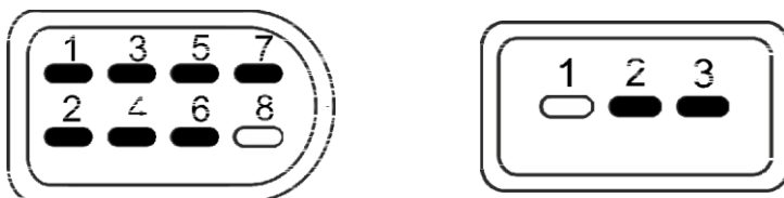
Рисунок 18. Разъем ТНВД тип 5: а – подача и индуктивный датчик, б – клапан опережения
