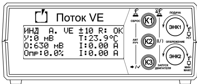
Рисунок 1. Панель передняя
