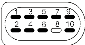
Рисунок 16. Разъем ТНВД тип 4
