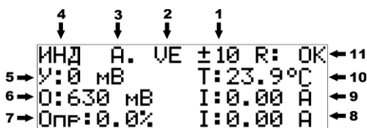
Рисунок 3. Описание информации на индикаторе прибора режим VE
