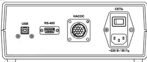
Рисунок 2. Панель задняя
