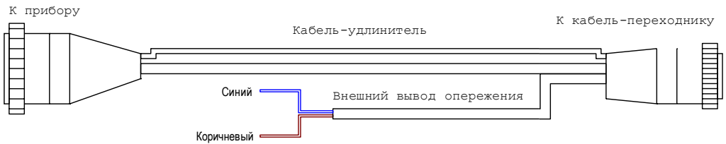
Рисунок 21. Кабель-удлинитель
