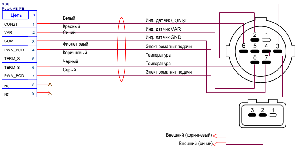
Рисунок 13. Схема распиновки разъема THVD тип 2
