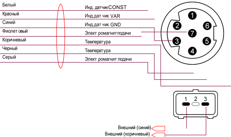
Рисунок 15. Схема распиновки разъема ТНВД тип 3
