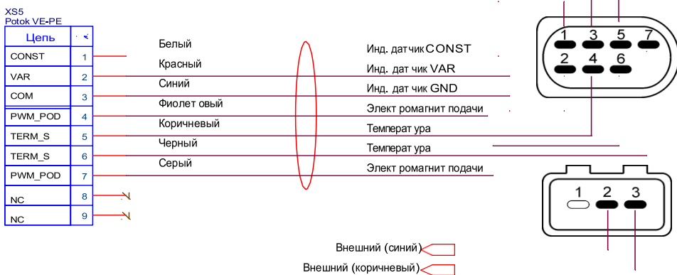
Рисунок 11. Схема распейки разъема ТНВД тип 1
