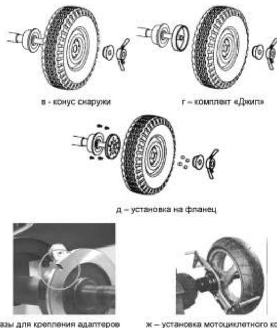
Рисунок 5.1 – Установка колеса
