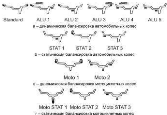
Рисунок 5.6 – Схемы установки грузов
