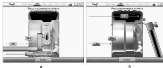
Рисунок 5.5 – Экран при втором измерении
