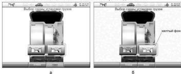
Рисунок 5.7 – Выбор схемы установки грузов
