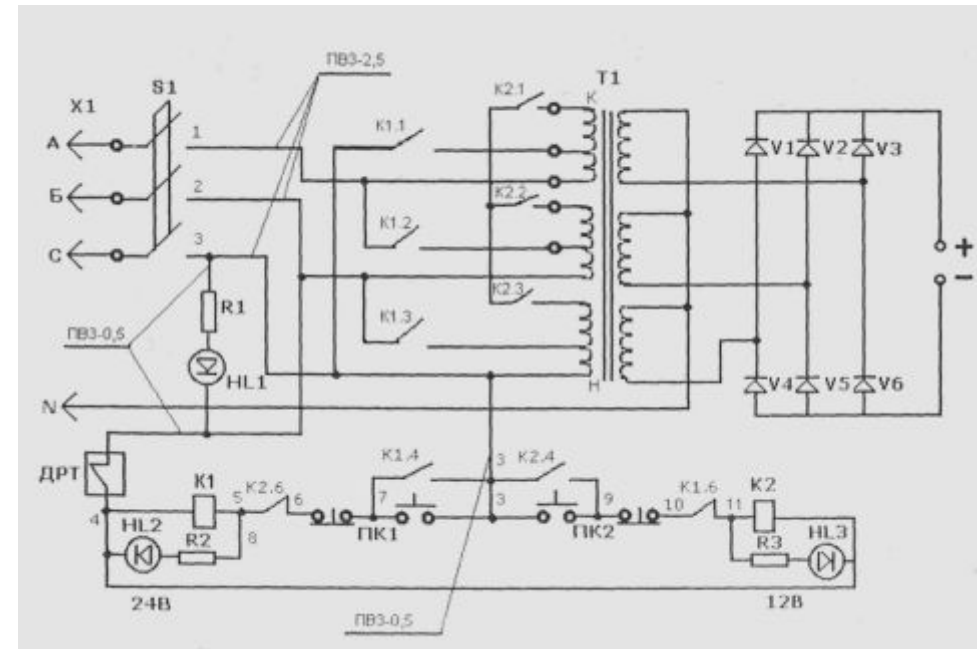
Рис.2. Схема электрическая принципиальная
