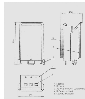
Рис.1 Общий вид пусковой установки
