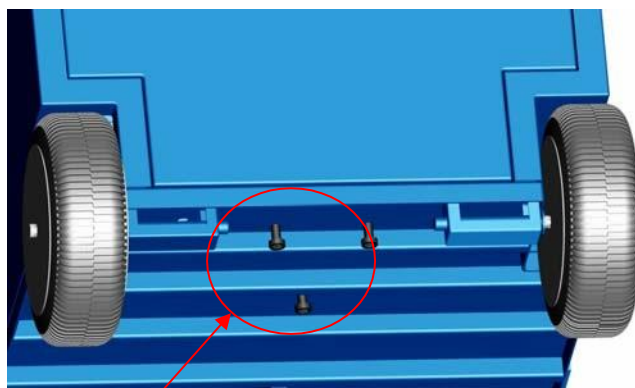
Три транспортировочных винта электронных весов
