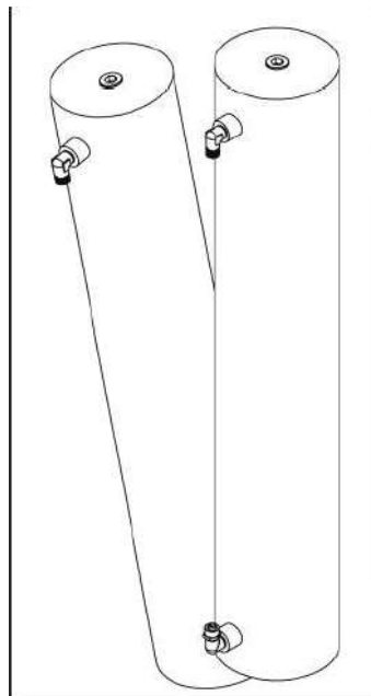
Рис. 5 Высокоэффективный фильтр-масловлагодетель (опция)
