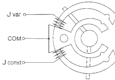
Рисунок 17. Индуктивные датчики положения рейки
