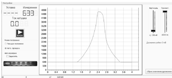
Рисунок 12. График проверки перемещения рейки насоса в автоматическом режиме на исправной централизации ZEXEL
