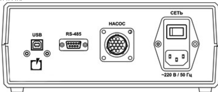
Рисунок 2. Панель задняя
