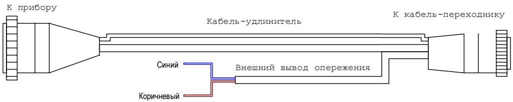
Рисунок 18. Кабель-удлинитель
