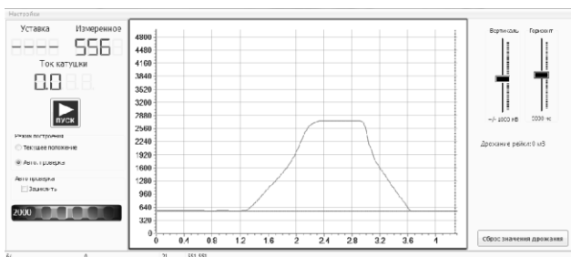
Рисунок 13. График проверки перемещения рейки насоса в автоматическом режиме на неисправной централизации ZEXEL
