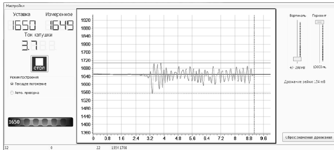
Рисунок 11. График дрожания рейки
