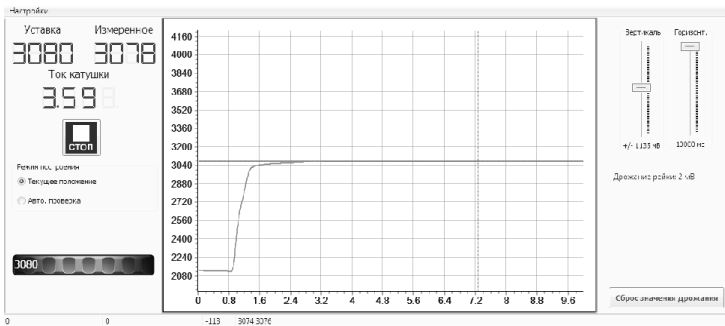
Рисунок 10. График нормально работающего насоса
