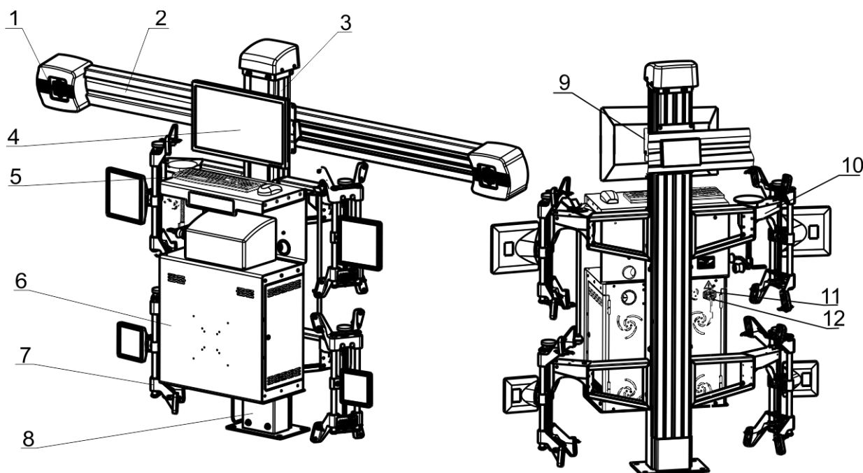
Рисунок 4.2 – Общий вид станда с кабинетом оператора консольным (ТЛ2ПС, М2ПС)
