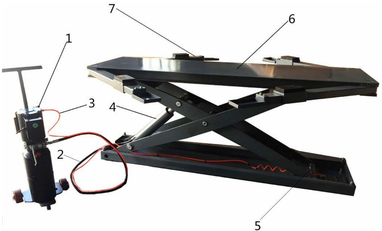
Рисунок 1. Комплектация ножничного подъемника «Siver Lift 1.30HMM»:
