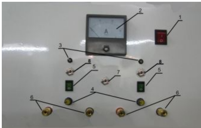
Рис. 1 Общий вид.
