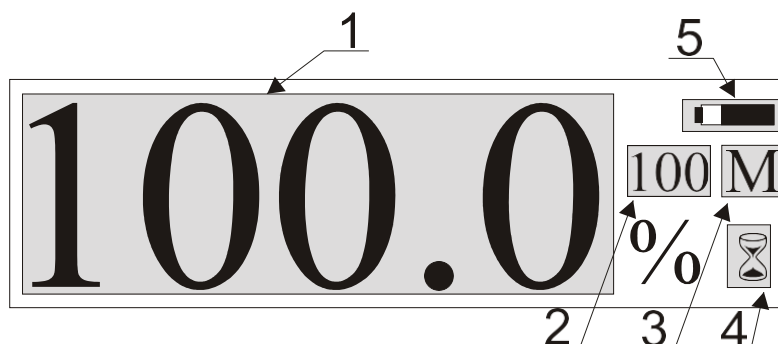
Рис. 5.3. ЖК индикатор прибора. 1 - значение коэффициента светопропускания, 2 - индикатор выполняемой задачи (измерение/установка 100%), 3 - индикатор запуска задачи (M - запуск с клавиатуры, С - с компьютера), 4 - индикатор хода выполнения задачи, 5 - индикатор заряда аккумулятора.
