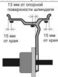
Рисунок 5.12 – Дистанции установки ленточных грузов
