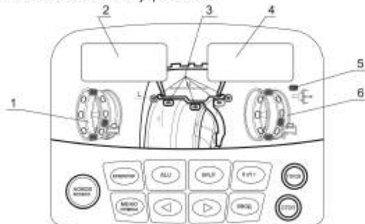
1, 6 – индикаторы положения груза; 2, 4 – цифровые индикаторы, 3 – индикатор схемы расположения грузов, 5 – индикатор режима компенсации адаптера
