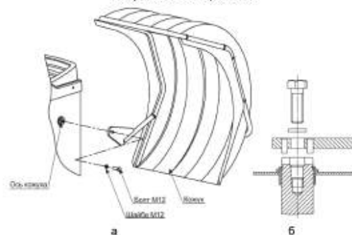
Рисунок 4.3 – Установка кожуха
