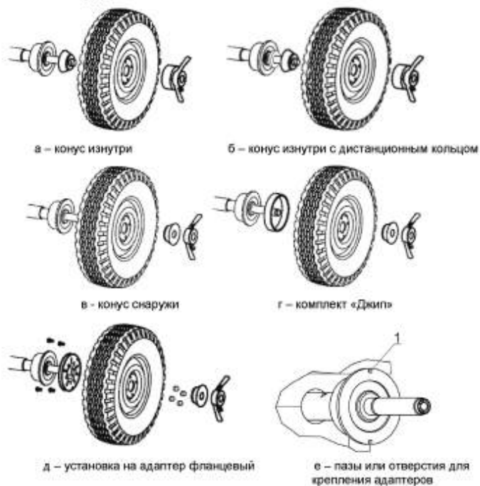
Рисунок 5.1 – Установка колеса
