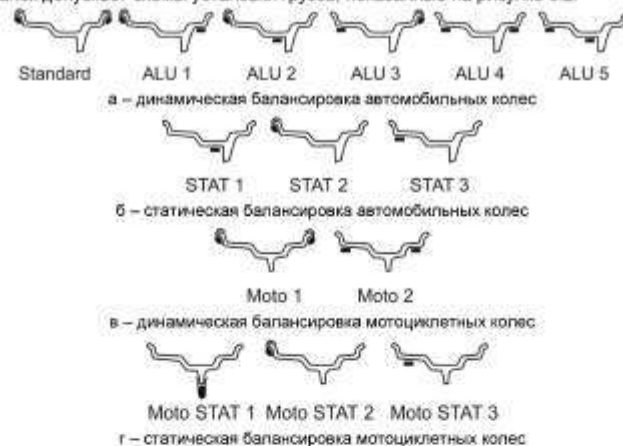
Рисунок 5.2 – Схемы установки грузов
