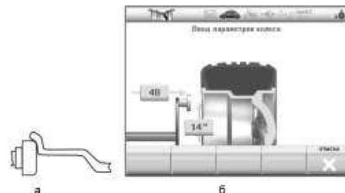
Рисунок 5.11 – Измерение электронной линейкой
