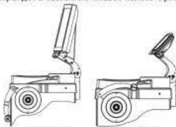
а – SBMP-40 Л б – SBMP-40 Ст Рисунок 4.7 – Исходное положение линейки
