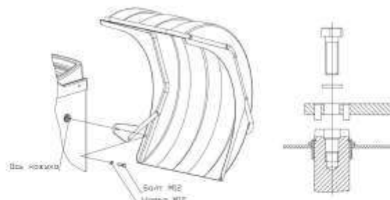
г – установка кожуха
