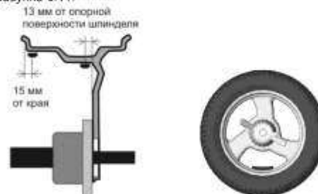
Рисунок 6.11 – Установка ленточных грузов
