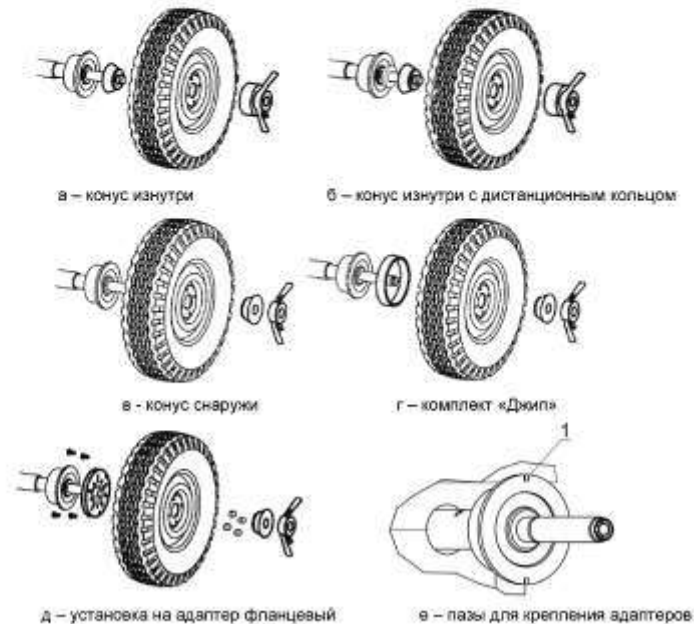
Рисунок 5.1 – Установка колеса
