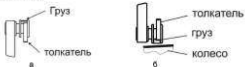
Рисунок 5.19 – Установка груза линейкой
