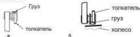
Рисунок 6.7 – Установка груза линейкой
