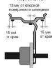
Рисунок 5.16 – Дистанции установки ленточных грузов вручную
