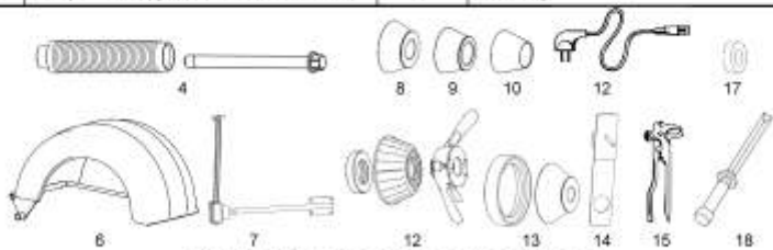
Рисунок 3.1 – Поставляемые принадлежности
