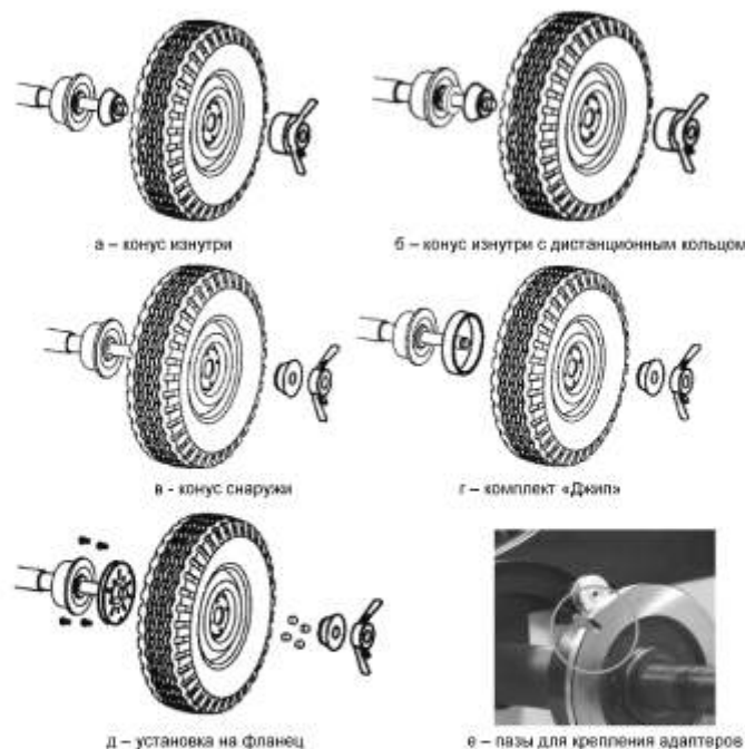
Рисунок 6.1 – Установка колеса
