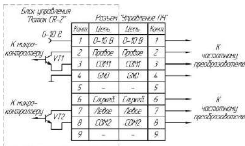
Рисунок 7.35 – Распайка разъема "Управление ПЧ".
