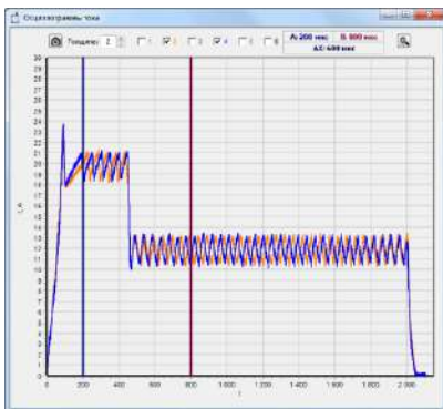
Рисунок 7.14 – Окно просмотра осциллограмм тока
