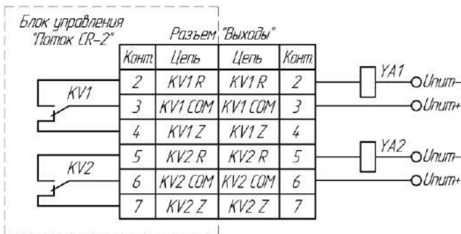
Рисунок 4.15 - Управление шторкой-задвижкой. Схема 3
