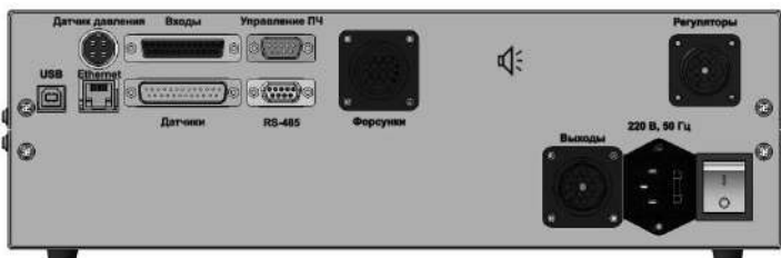
Рисунок 1.3 – Задняя панель
