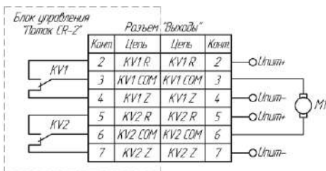
Рисунок 7.30 - Управление шторкой-задвижкой. Схема 1
