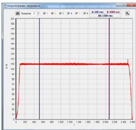
Рисунок 7.15 – Окно просмотра осциллограмм напряжения
