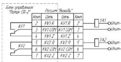
Рисунок 7.32 - Управление шторкой-задвижкой. Схема 3
