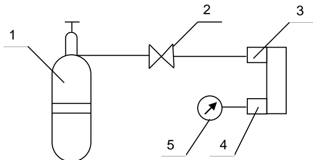
Рис.3.Схема проверки герметичности газового тракта
